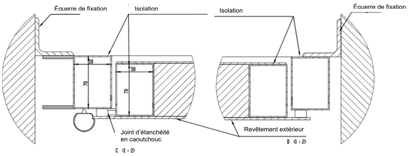
Exemple vue AQUALOCK porte – version isolée – Profils simplifié
