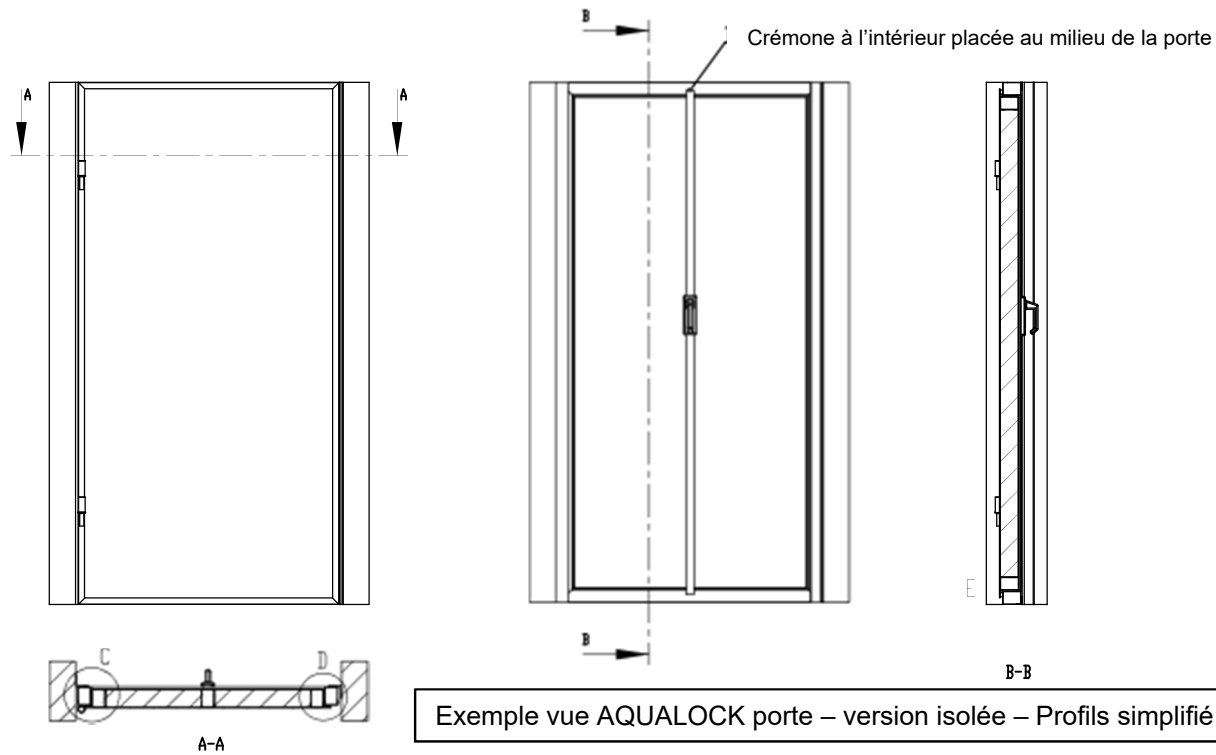
Exemple vue AQUALOCK porte – version isolée – Profils simplifié
